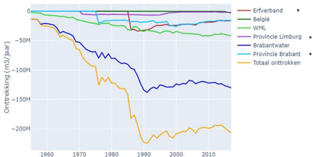
Figuur 4.2 Omvang diepe grondwateronttrekkingen Centrale Slenk door verschillende partijen, 1955-2020
